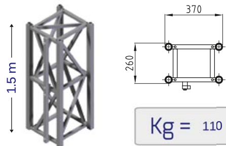
Traliccio quadrato Square mast - Mât carré
